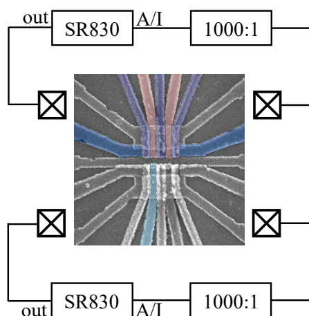
图 3.9 量子点输运的粗测线路主要由锁相放大器和高精度直流电源构成。其中，锁相放大器的输出端 A/I 通过 1000:1 的分压连接到量子点的源极，输入端 out 连接在量子点的漏极；高精度直流电源用于为各个电极提供稳定的直流偏置电压，相关连接在示意图中未作详细绘出。
