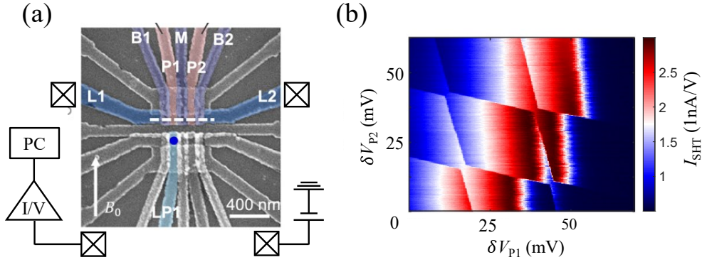
图 3.12 (a) 量子点直流测量线路示意图，主要使用到的仪器是高精度直流源以及放大器。(b) 直流测量的双量子点相图，图中的本底代表单空穴晶体管的库仑峰，库仑峰之上叠加的突变信号为量子点中空穴的隧穿信号。
