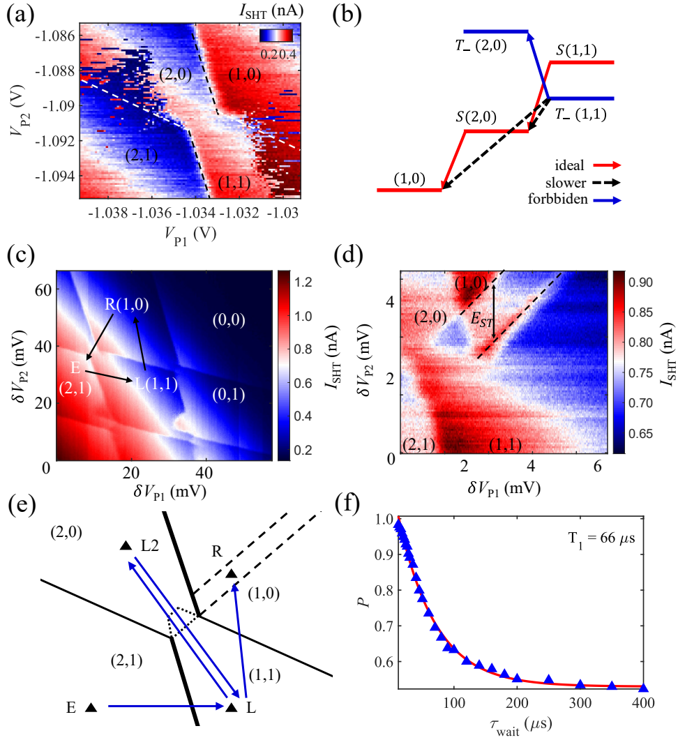
图 5.6 (a) 不同源漏隧穿速率的双量子点相图, P1 电极下的量子点的隧穿线信号集中且清晰, P2 电极下量子点的隧穿线信号松散且微弱, 这说明双量子点与源漏的隧穿速率不同。(b) 在 (1,1) - (2,0) 区域附近的能级示意图。(c) (1,1) - (2,0) 区域的能级图, 图中展示的是增强型锁存读取所采用的 E(2,1) - L(1,1) - R(1,0) 三段波形。(d) 增强型锁存读取的区域由黑色虚线标出, 两个虚线之间距离为三重态和单重态之间的能量差 E_{\text{ST}} 。(e) 测量 (1,1) 区域的自旋弛豫时间 T_1 采用五阶段波形序列。(f) 单重态概率 P 呈指数衰减, 拟合该衰减曲线可提取到自旋弛豫时间 T_1 = 66 \mu\text{s} 。
