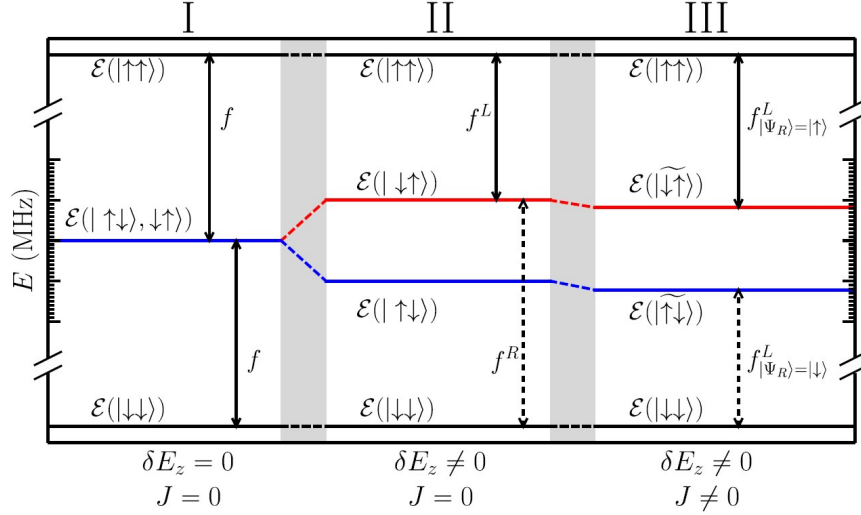
图 2.5 两个自旋在存在磁场梯度的双量子点中的本征能量 E ，以及在三种不同参数区域下它们之间的相关跃迁。区域 I 描述的是没有磁场梯度的情况，此时单自旋翻转跃迁在能量上是简并的。区域 II 表示在存在磁场梯度时，左侧自旋与右侧自旋之间的跃迁频率简并被打破，从而可以从能量上区分对左自旋和右自旋的单比特操作。进一步打开交换相互作用 J （区域 III），左侧自旋的共振频率会依赖于右侧自旋的状态，因此可以通过频率选择实现两比特门操作。图源自 [137] 。
