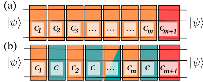
图 2.7 随机基准测试中的两种实验序列 (a) 标准基准测试序列示意图。 C_1 - C_m 是随机从 Clifford 门中选取的 m 个门操作。执行最后的 C_{m+1} (红色) 以使总序列等于恒等操作。(b) 交错基准测试序列的示意图, C (绿色) 与从 Clifford 中选择的随机门 C_i (橙色) 交错, 执行最后的门 C_{m+1} (红色) 以使总序列等于恒等操作。图源自 [143] 。
