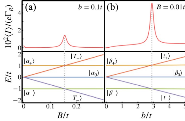
图 4.4 (a) 施加面内磁场时, 双量子点 g 因子差异引起的漏电流随外磁场的变化。下方为能级示意图, 当三重态 |T_{\pm}\rangle 与 S(1, 1) 和 S(2, 0) 的叠加态 |\alpha_{\pm}\rangle 发生共振时, 对应磁场下出现电流峰。(b) 施加面外磁场时, 双量子点 g 因子差异引起的漏电流随外磁场的变化。当三重态 |t_{\pm}\rangle 与 S(1, 1) 和 S(2, 0) 的叠加态 |\beta_{\pm}\rangle 发生共振时, 对应磁场下出现电流峰图源自 [168]。
