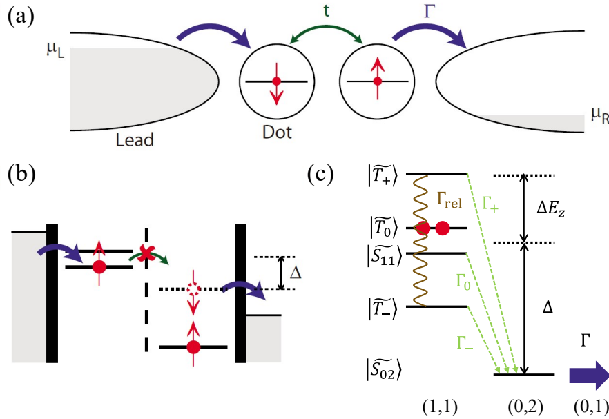
图 4.7 (a) 双量子点与左右两个引线电极耦合, 由于源漏的偏置电压, 电子只能从左侧电子库流向右侧电子库。(b) 在隧穿保自旋的情况下, 只有 S(1, 1) 态能够到达 S(0, 2) 态。 T(1, 1) 态不能隧穿到 S(0, 2) 态, 电流被阻塞。(c) 假如可以发生自旋翻转隧穿, 考虑高磁场并且忽略核自旋的影响, 四个 (1, 1) 态中有三个可以弛豫到 S(0, 2) 态, 从而出现漏电流。其中 \Delta 为 (1, 1) 电荷配置中 S 态和 T 态之间的能量差, \Delta E_z 为塞曼劈裂能。图源自 [169] 。
