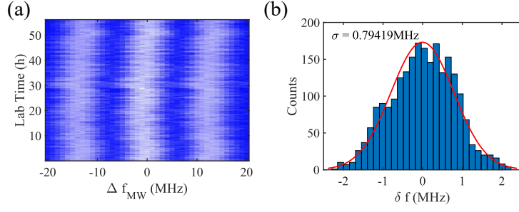
图 5.16 (a) 固定等待时间 \tau_{\text{idle}} = 40 \text{ ns} , 在 55h 内测得的 Ramsey 实验结果 (b) 对 55h 内的比特频率抖动进行统计分析, 发现其呈现出近似高斯分布, 其标准差为 0.794 MHz。
