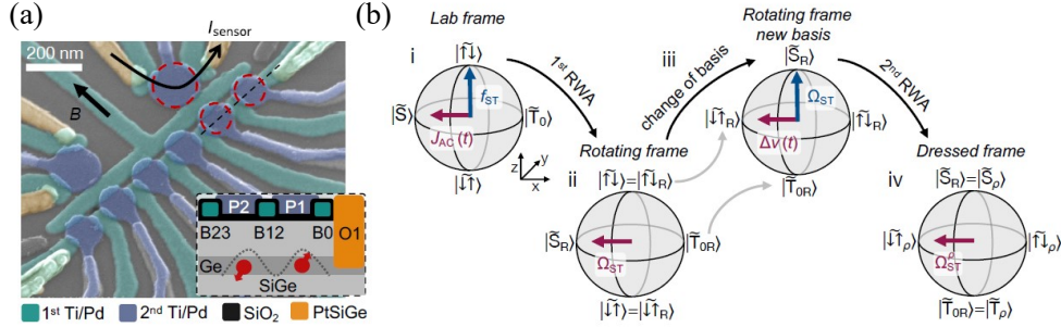
图 5.1 (a) IBM 团队开展缀饰态单重态三重态量子比特实验使用的六量子点器件的扫描隧道显微镜照片。(b) 通过每个阶段的布洛赫球逐步展示说明缀饰态量子比特的操作过程。图片摘录自文献 [233]
