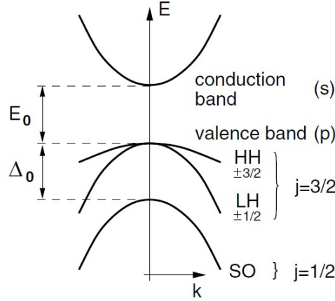
图 4.6 自旋-轨道相互作用导致最上方价带发生分裂, 劈裂的能量差为 \Delta_0 。由于应力或者缺陷的影响, j = 3/2 的价带会进一步劈裂成为重空穴带与轻空穴带。图源自 [225] 。
