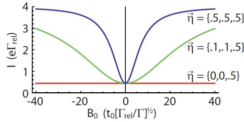
图 4.8 自旋轨道相互作用引起的漏电流磁谱, 随着磁场的增大, 三重态发生劈裂并发生态杂化, 有一定的概率转移到 S(0, 2) 态, 从而产生漏电流。所以漏电流磁谱表现为 0 磁场附近的谷, 并且谷的半高宽代表了自旋轨道耦合相互作用的强度, \vec{\eta} 代表三维磁场方向上的自旋轨道相互作用强度。图源自 [169] 。
