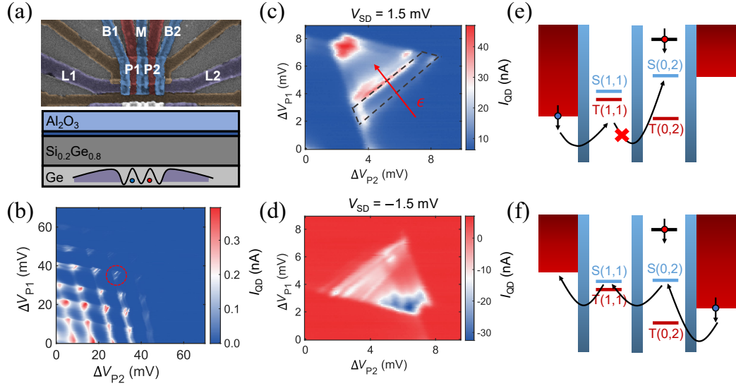
图 4.1 (a) 平面锗双量子点器件的伪彩色扫描电子显微镜 (SEM) 图像以及栅极下方简化衬底结构的截面示意图。(b) 施加源漏偏压之后的双量子点相图, 可以观察到一系列的偏压三角形。红色虚线圆圈圈出的为后续发现泡利自旋阻塞的位置, 大致的空穴数为 6。(c-d) \pm 1.5 \text{ mV} 下的偏压三角形, 对比两个三角形发现, 二者大小相近, 但是正偏压三角形的底部存在一块输运电流缺失的梯形区域, 此处为泡利自旋阻塞区域。红色箭头代表双点失谐的正方向。(e-f) 泡利自旋阻塞的能级及其物理机制示意图。
