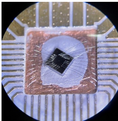
图 3.8 用银胶贴片在 PCB 板上的量子点芯片，芯片引脚与 PCB 板通过铝线键合。
