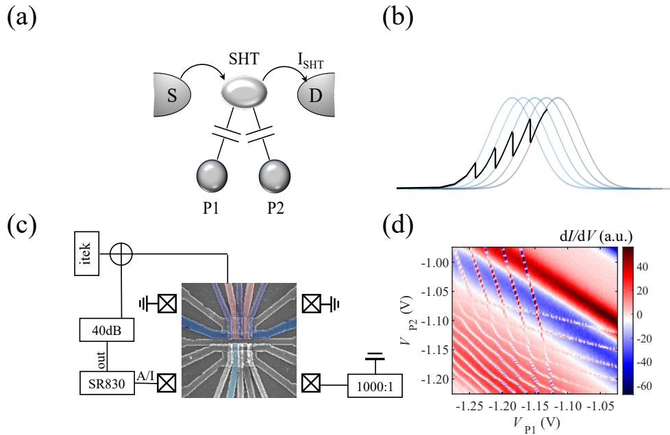
图 3.11 (a) 单空穴晶体管与量子点电极之间的电容耦合示意图，图源自 [16] 。(b) 量子点中空穴数变化对于单空穴晶体管电流峰的影响。(c) 量子点调制测量的实验电路示意图。(d) 调制测量得到的双量子点相图，可以清晰地分辨出两组互相交叉的平行隧穿线，相图的右上角不再有隧穿线出现说明双量子点可以被耗尽到最后一个空穴。
