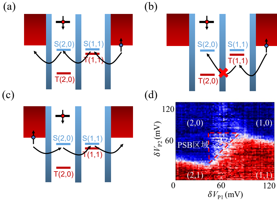
图 5.5 (a-c) 不同点间失谐情况下, 单重态 S 与三重态 T 的隧穿情况, a-b 图中在失谐小于 E_{ST} , 若形成的是 S(1, 1) , 空穴可以在双点之间自由隧穿, 若形成的是 T(1, 1) , 空穴的隧穿被阻塞。c 图中在失谐大于 E_{ST} , 即使形成原本被阻塞的三重态 T , 空穴也能够发生隧穿。(d) (1, 1) - (2, 0) 区域的泡利自旋阻塞区域, 图中使用红色虚线围起的三角形区域为泡利自旋阻塞区。
