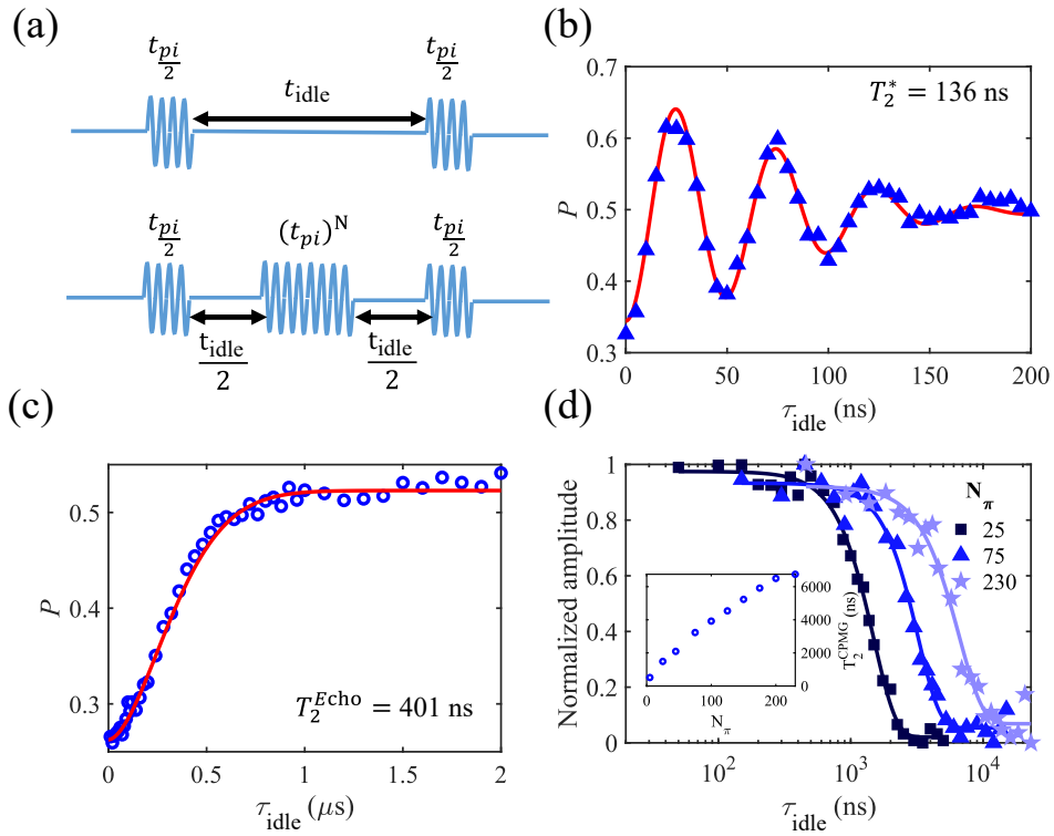
图 5.8 (a) 拉姆齐实验与 CPMG 实验 ( N=1 时为哈恩回波实验) 的微波波形序列示意图。(b) 比特频率 10 MHz 失谐情况下的拉姆齐实验的结果，拟合得到退相位时间 T_2^* = 136 ns。(c) 哈恩回波实验的结果，拟合得到相干时间 T_2^{\text{Echo}} = 401 ns。(d) CPMG 实验中不同阶数的 N_\pi 下得到的相干时间 T_2^{\text{CPMG}} 。给出了 N_\pi = 25, 75, 230 条件下的 CPMG 测量结果。
