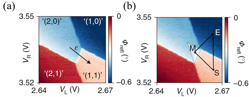
图 2.4 (a) 所关注区域的电荷稳定性图。每个库仑阻塞区域内的有效空穴占据数以“(NL, NR)”表示，其中引号表示等效空穴数。实际占据数满足：NL 为 3 或 4（取决于具体阻塞区间），NR 为 2n 或 2n + 1 ( n 为整数)。对角箭头标示的是失谐 \epsilon 的调控方向。(b) 该稳定性图是在沿箭头所示顺时针路径施加脉冲时测得。系统首先在 (1, 0) 处被初始化(E)，随后跃迁至 (1, 1) ，此时可形成单重态或三重态。进一步脉冲至 (2, 0) 的测量点(M)后，三重态因泡利阻塞而无法完成跃迁，从而在图中形成特征性的三角形阻塞区域。图源自 [131]
