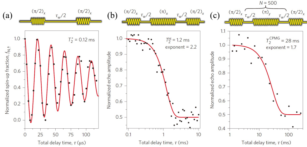
图 2.6 (a) Ramsey 实验波形示意图以及实验结果，通过改变两个 \pi_x/2 脉冲之间的延迟时间 \tau_w ，在自旋向上概率 f_{\uparrow} 中出现 Ramsey 振荡，拟合得到相干时间 T_2^* = 120 \mu\text{s} 。(b) Hahn-Echo 实验波形示意图以及实验结果。在 Ramsey 波形的基础上加入了一个额外的 \pi 脉冲，拟合得到相干时间 T_2^H = 1.2 \text{ ms} 。(c) CPMG 脉冲序列是在两个 \pi_x/2 脉冲之间加入多个 \pi_y 操作，进一步增强相干时间，得到 T_2^{\text{CPMG}} = 28 \text{ ms} 。图源自 [51] 。
