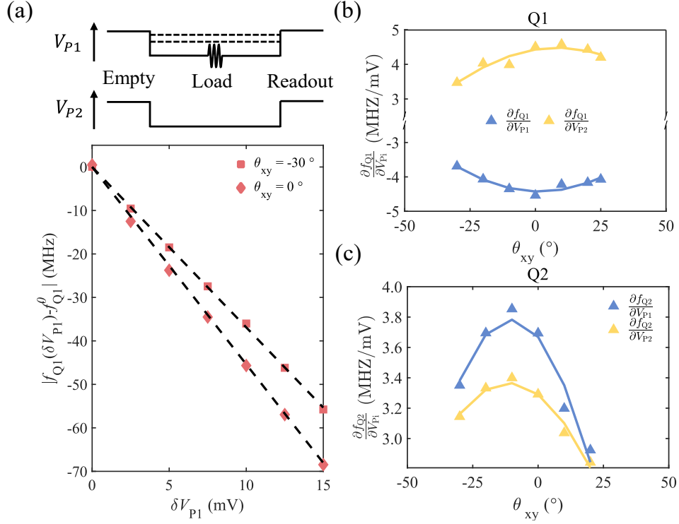
图 6.3 (a) 图上半部分为测量纵向自旋-电场敏感度 (LSES Q1 和 LSES Q2 ) 所采用的脉冲序列。该序列包含三个阶段——Empty、Load 和 Readout——分别对应电荷构型 (1, 0)、(1, 1) 和 (1, 0)。量子比特操控在 Load 阶段进行。通过改变施加在调节栅极 P1 或 P2 上的电压, 可以相应调制量子比特 Q1 和 Q2 的共振频率。由此提取量子比特频率随栅压变化的偏移量, 并绘制于 (a) 的下半部分中。频率偏移与所施加的栅电压呈线性关系, 由其斜率即可得到 LSES。图中展示了在磁场方向 \theta_{xy} = -30^\circ 和 \theta_{xy} = 0^\circ 时测得的 LSES P1 的代表性结果。(b-c) 量子比特 Q1 和 Q2 的 LSES 随面内磁场角度 \theta_{xy} 的变化关系。对于量子比特 Q1, 来自栅极 P1 (蓝色三角) 和 P2 (黄色三角) 的 LSES 既有正值也有负值, 表明两个栅极对 Q1 的影响方向相反。 \frac{\partial f_{Q1}}{\partial V_{P1}} 和 \frac{\partial f_{Q1}}{\partial V_{P2}} 均随 \theta_{xy} 呈现明显的抛物线型变化, 并在 \theta_{xy} = 0^\circ 处达到最大值。当磁场方向偏离该角度时, LSES Q1 逐渐减小, 反映出自旋-电场敏感度减弱以及电荷噪声导致的退相干受到抑制。量子比特 Q2 也表现出类似的角度依赖行为。值得注意的是, \frac{\partial f_{Q2}}{\partial V_{P1}} (蓝色三角) 大于 \frac{\partial f_{Q2}}{\partial V_{P2}} (黄色三角)。这一现象归因于两个独立量子点与源漏之间存在不对称隧穿速率, 使得位于 P1 下方的量子点受到更强的“压缩”, 变化 P1 电压对于双量子点的限制势影响更大。在整个角度范围内, LSES Q2 始终保持为正值, 说明施加在 P1 和 P2 上的电压都会增强 Q2 的面内 g 因子。LSES Q2 的最大值出现在 \theta_{xy} = -10^\circ 处。
