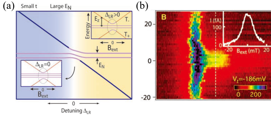
图 4.3 (a) 在小的双点隧穿耦合 ( t )，大的 Overhauser 场情况下，在整个双点失谐 (detuning, \Delta_{LR} ) 范围内， T(1,1) 和 S(1,1) 发生显著混合。(b) 在小的双点隧穿耦合 ( t )，大的 Overhauser 场情况下，漏电流随外磁场 ( B_{\text{ext}} ) 单调下降，形成一个关于 0 磁场对称的电流峰。图源自 [221] 。
