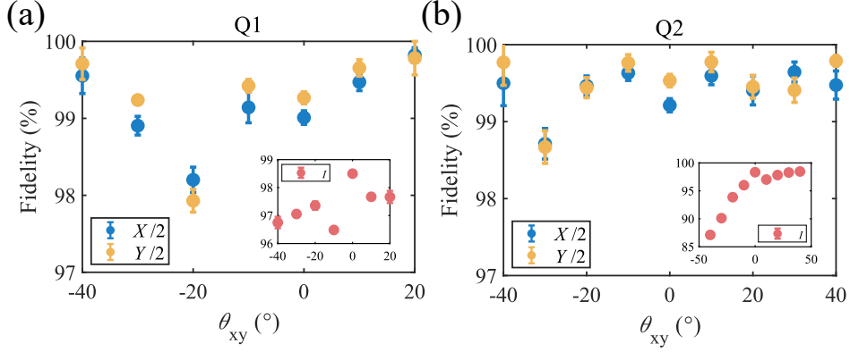
图 6.7 (a-b) 门操作集合 I/2 、 X/2 、 Y/2 的控制保真度随面内磁场角度 \theta_{xy} 的变化关系。 X/2 和 Y/2 门的保真度随 \theta_{xy} 呈现非单调变化，即先降低后升高。最低保真度出现在 T_2^{\text{Echo}} 最短的磁场方向处。对于量子比特 Q1 (Q2)，最佳控制保真度相较于最差情况分别提升约 2% (1%)，并且均超过量子计算容错阈值。 I 门的保真度同时依赖于 T_2^* 和 f_{\text{Rabi}} 。由于在整个 \theta_{xy} 扫描范围内 T_2^* 基本保持不变，因此 I 门保真度主要由 f_{\text{Rabi}} 决定 [328] 。对于 Q1， I 门保真度随 \theta_{xy} 呈现非单调变化趋势，这与图 6.6 (a) 中 f_{\text{Rabi}} 的行为一致。对于 Q2，其保真度先随角度增加而提升，随后趋于饱和，同样遵循图 6.6 (a) 中 f_{\text{Rabi}} 的变化趋势。这种饱和现象表明，单纯提高 f_{\text{Rabi}} 对提升门保真度的作用逐渐减弱；若要进一步优化门保真度，还需要改善其他量子比特参数，例如 T_2^* 和 T_2^{\text{Rabi}} 等相干相关特性。误差棒代表 95% 置信水平。
