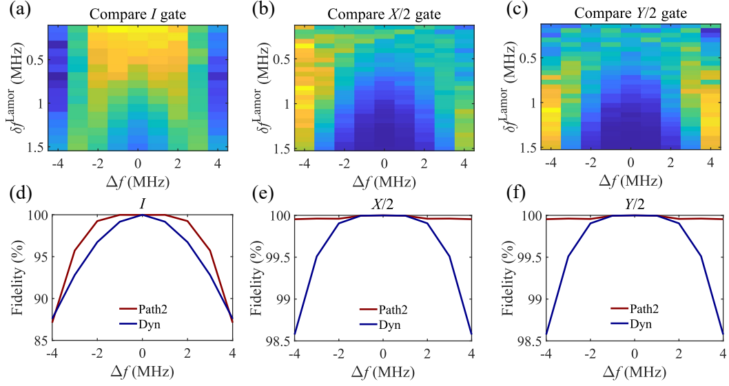
图 5.20 (a-c) 在不同的外加微波驱动频率失谐噪声 \Delta f 以及体系内在的比特频率抖动噪声 \delta f^{\text{Larmor}} ，几何量子门与传统动力学门操控保真度的差值。(d-f) 目前平面锗中最长的相干时间 17.6 \mu\text{s} ，估算得到 \delta f^{\text{Larmor}} = 0.012 \text{ MHz} 。数值模拟得到的几何门与传统动力学门保真度的差值。
